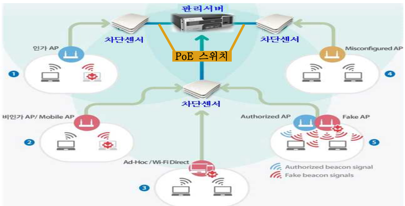
[그림] 무선침입차단시스템 구성도
