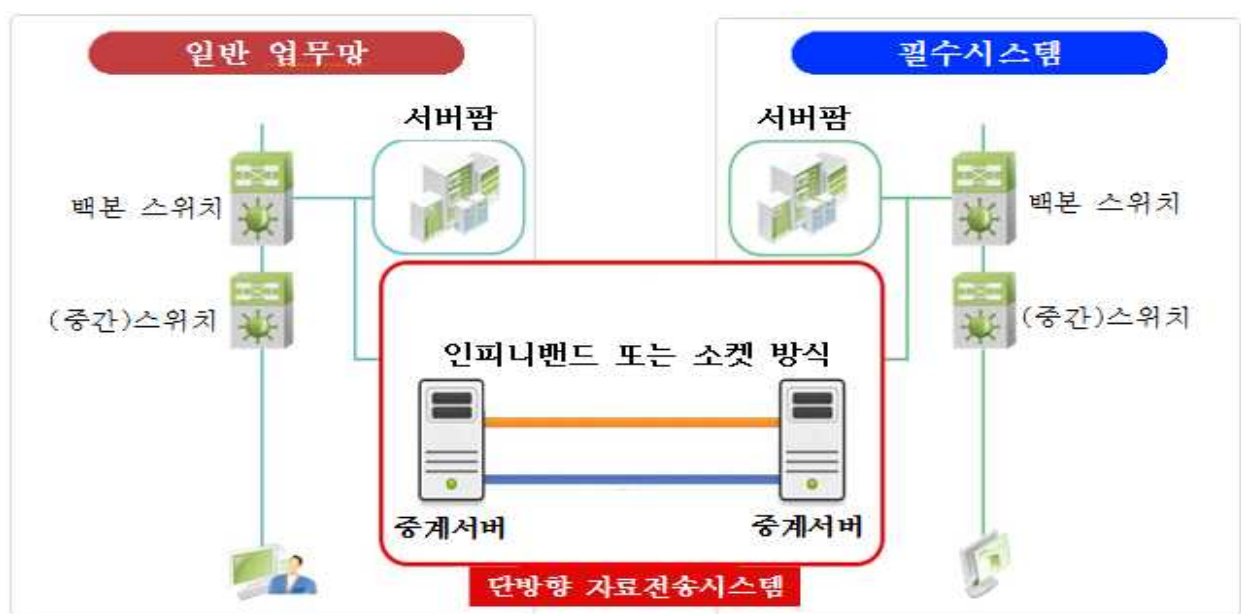
[그림 1] 단방향 자료전송시스템 구성도
