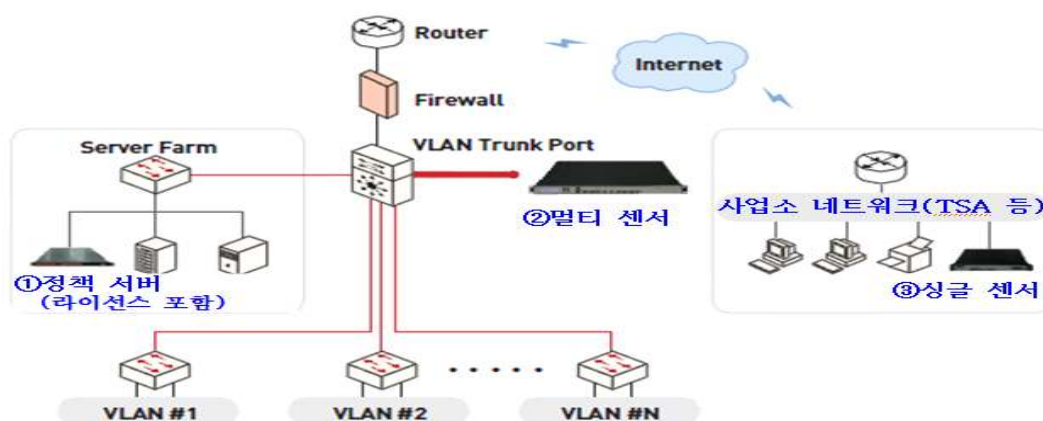
[그림 1] 네트워크 접근제어시스템 구성도
